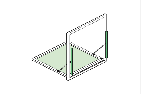
BILICO VERTICALE. Finestra a vasistas.
