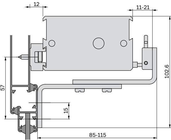
ESEMPIO DI INSTALLAZIONE 02 Installazione con staffa in plastica a coda di rondine (inclusa).
