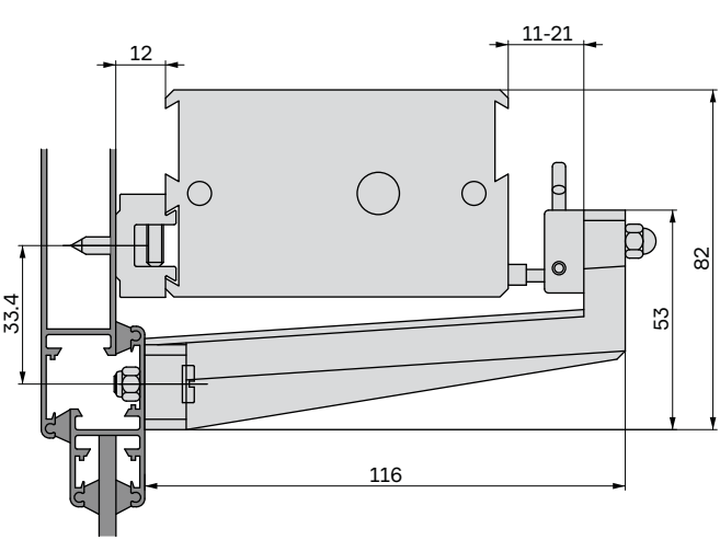
ESEMPIO DI INSTALLAZIONE 01 Installazione con staffa in plastica a coda di rondine (Inclusa).
