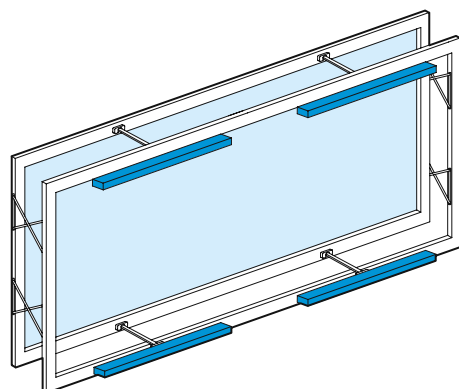
Finestra parallela.
