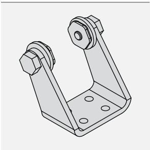
Staffa scorrevole
