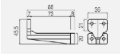
Staffa per finestra incernierata in alto (inclusa)
