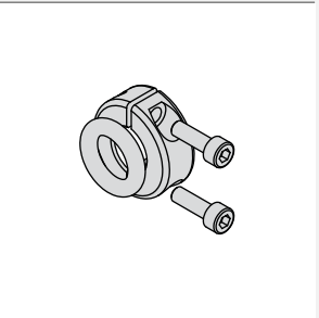
Kit di riduzione del corsa 40735V
