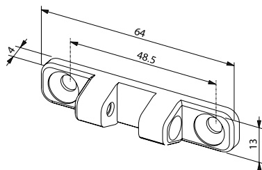
CONNECTOR CONNETTORE
